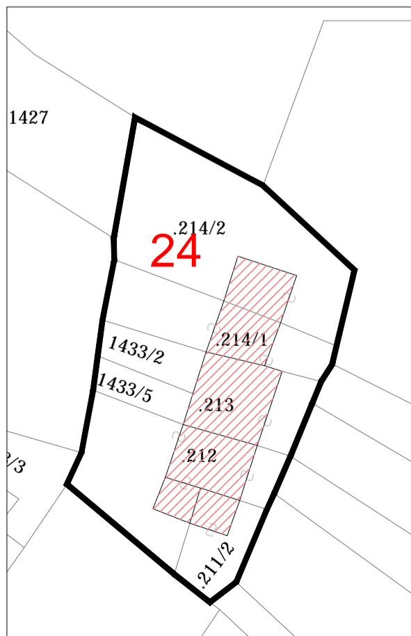
CENTRO STORICO ISOLATO N°24 - SCALA 1:500
